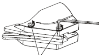
Рис 4 Стопорные винты
